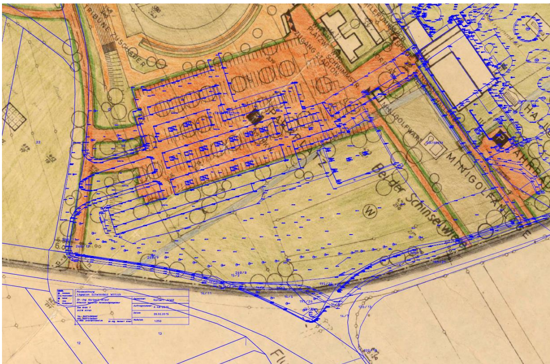
Abbildung 3: Überlagerung Vermessung (blaue Linien) und Ursprungsbebauungsplan
