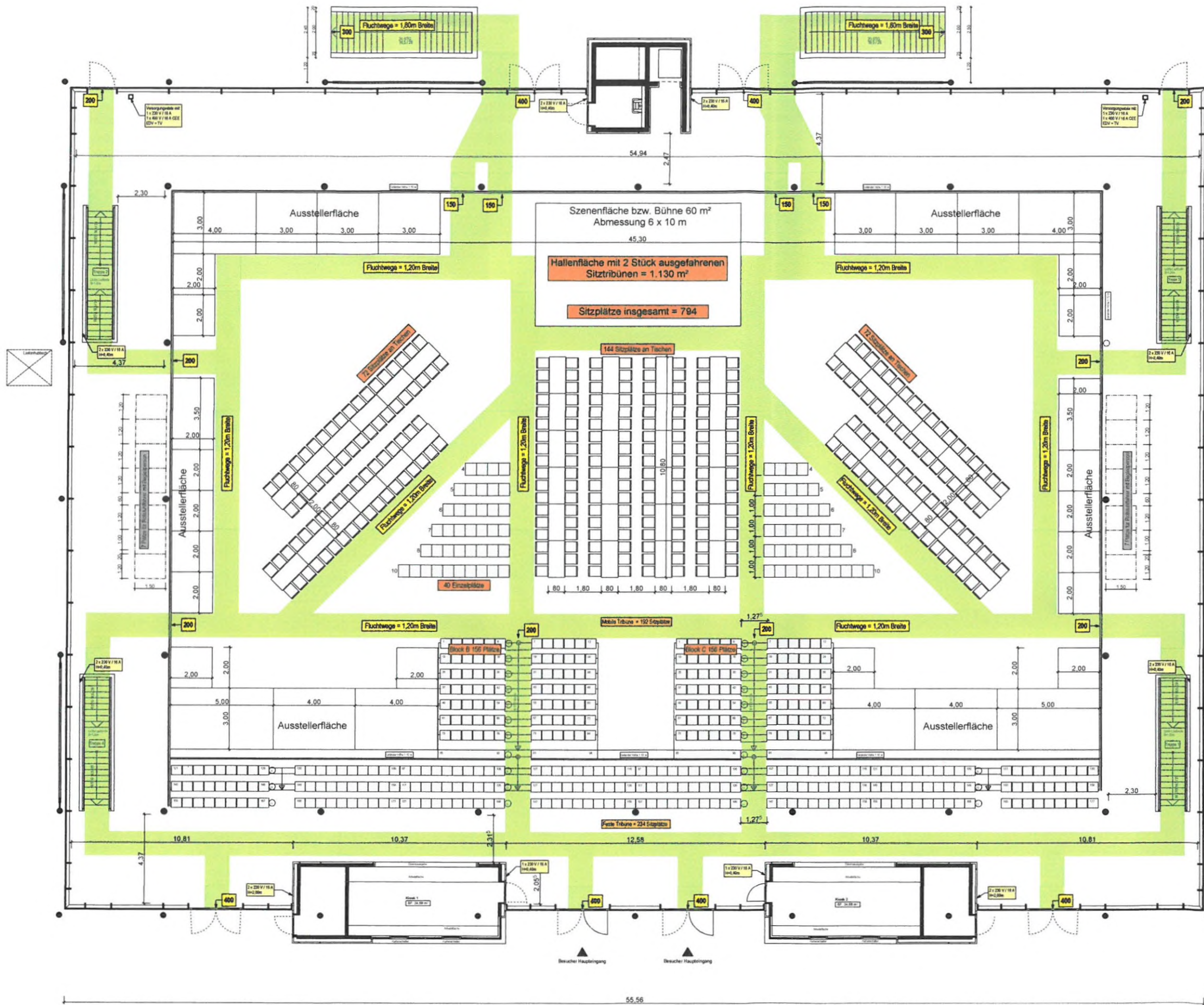
Grundriss Erdgeschoss
